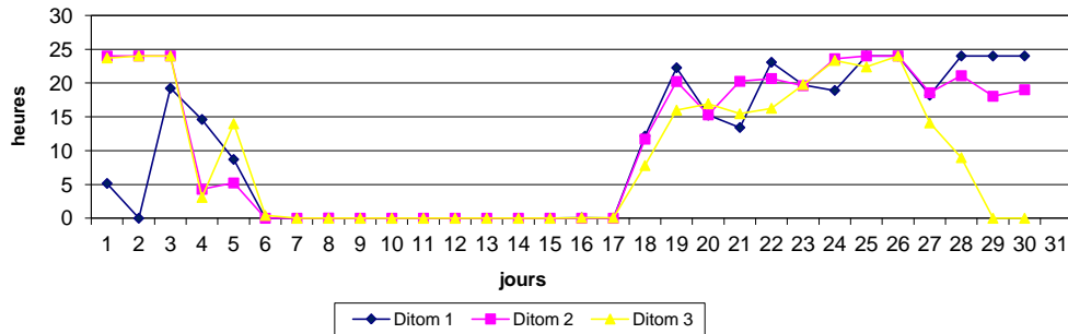
Evolution de la production électrique des moteurs à gaz
