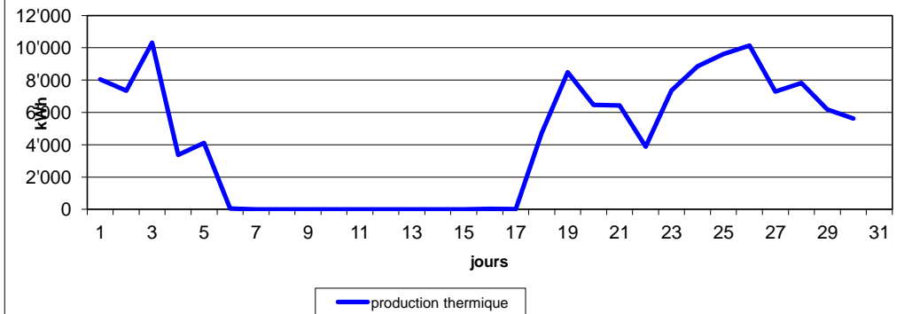
Evolution de l'énergie thermique produite
